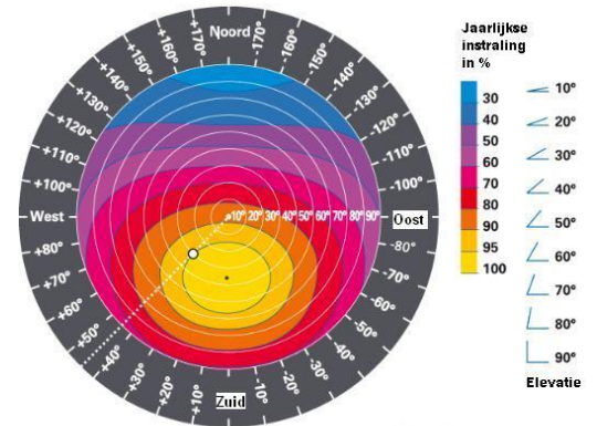
O : Voorbeeld: Elevatie 30 graden, Oriëntatie 45 gr ZuidWest is ongeveer 95%
